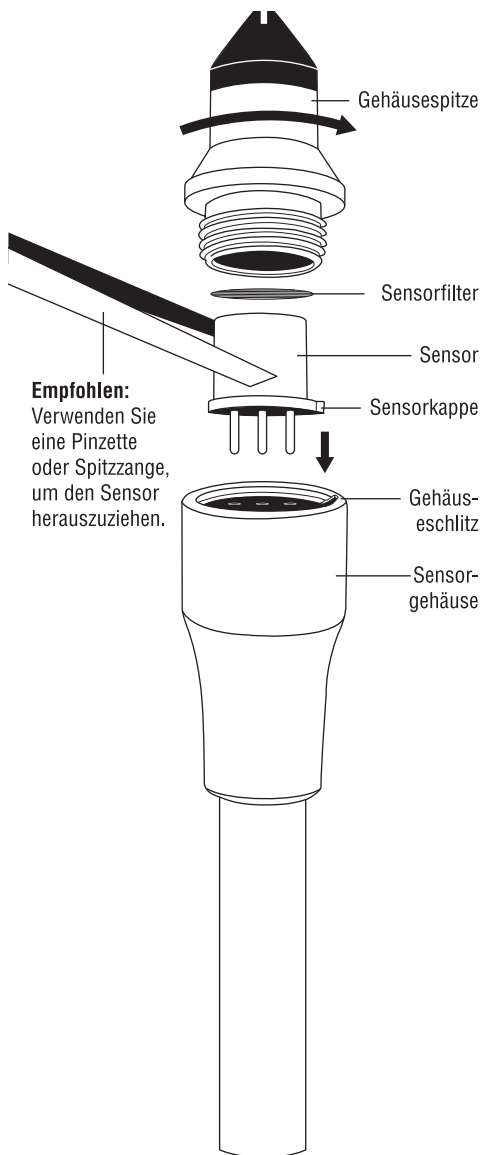
Abbildung: Sensoraustausch
